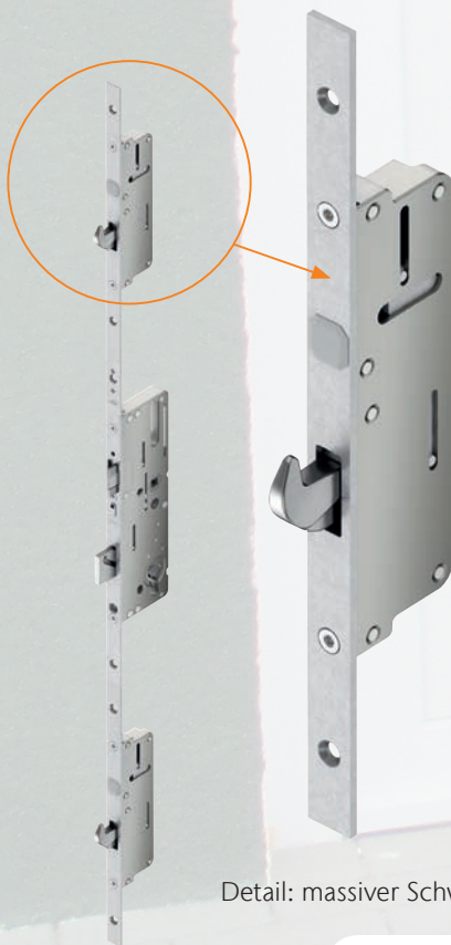
Schwenkriegelschloss
