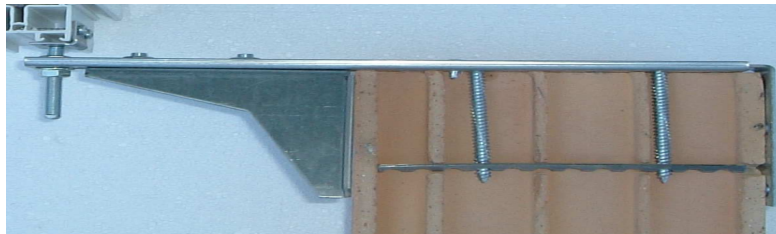
Ankerbefestigung am Hochlochstein mit der Lochschiene und Winkelsch.
