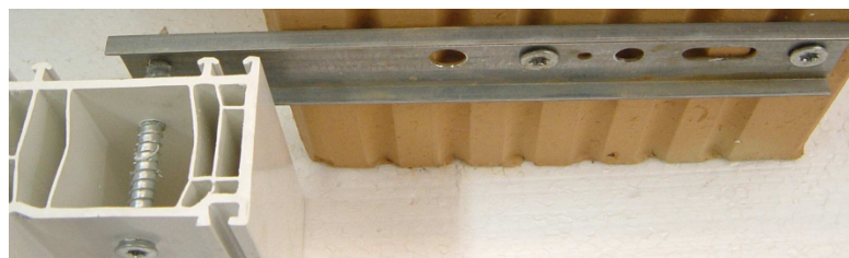
EL-Anker U-Profil als Verlängerung des Mauerwerkes
