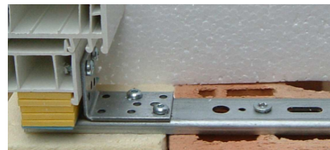
für die Verbindung zwischen Fenster und EL - Anker - Art.-Nr.: 405112
