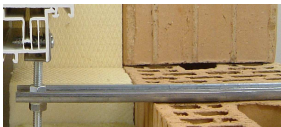
WU - Anker unten Kunststofffenster
