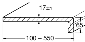
Blendenhöhe: 65 mm
