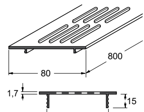
Lüftungsgitter
