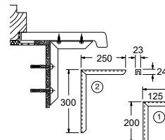
Konsolen
