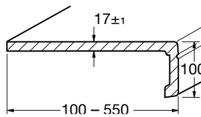
Blendenhöhe: 100 mm
