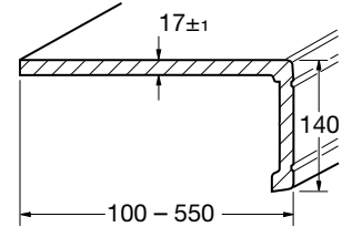
Blendenhöhe: 140 mm
