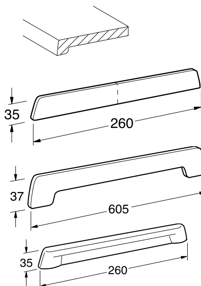
Seitenabschlusskappen für Innenfensterbänke
