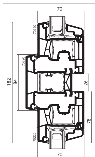
Profine KBE 70 zweiflügelig
