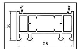
Blendrahmenverbreiterung
