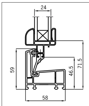
Profilquerschnitt isolierverglast 24 mm UG 1.1
