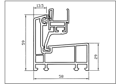
Kipp-Blendrahmen isolierverglast 14 mm
